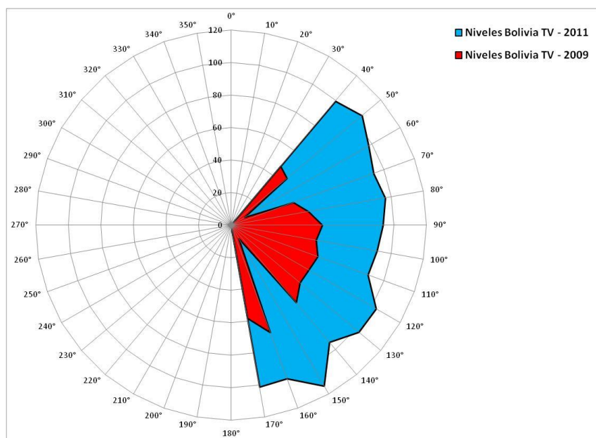
DIAGRAMA POLAR DISTANCIA 5 KM.
